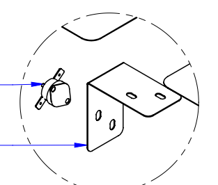
DETALHE U ESCALA 1 : 4
